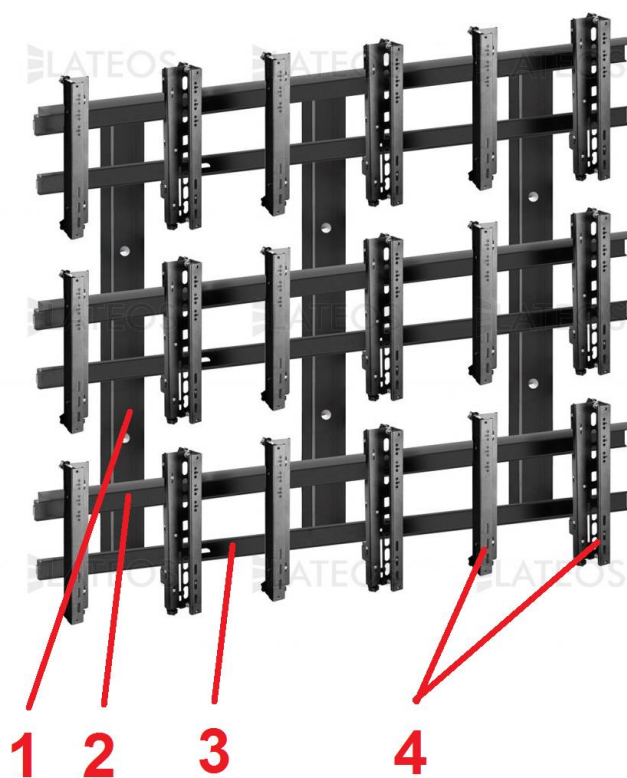
Рис.1 Кронштейн напольный в сборе
