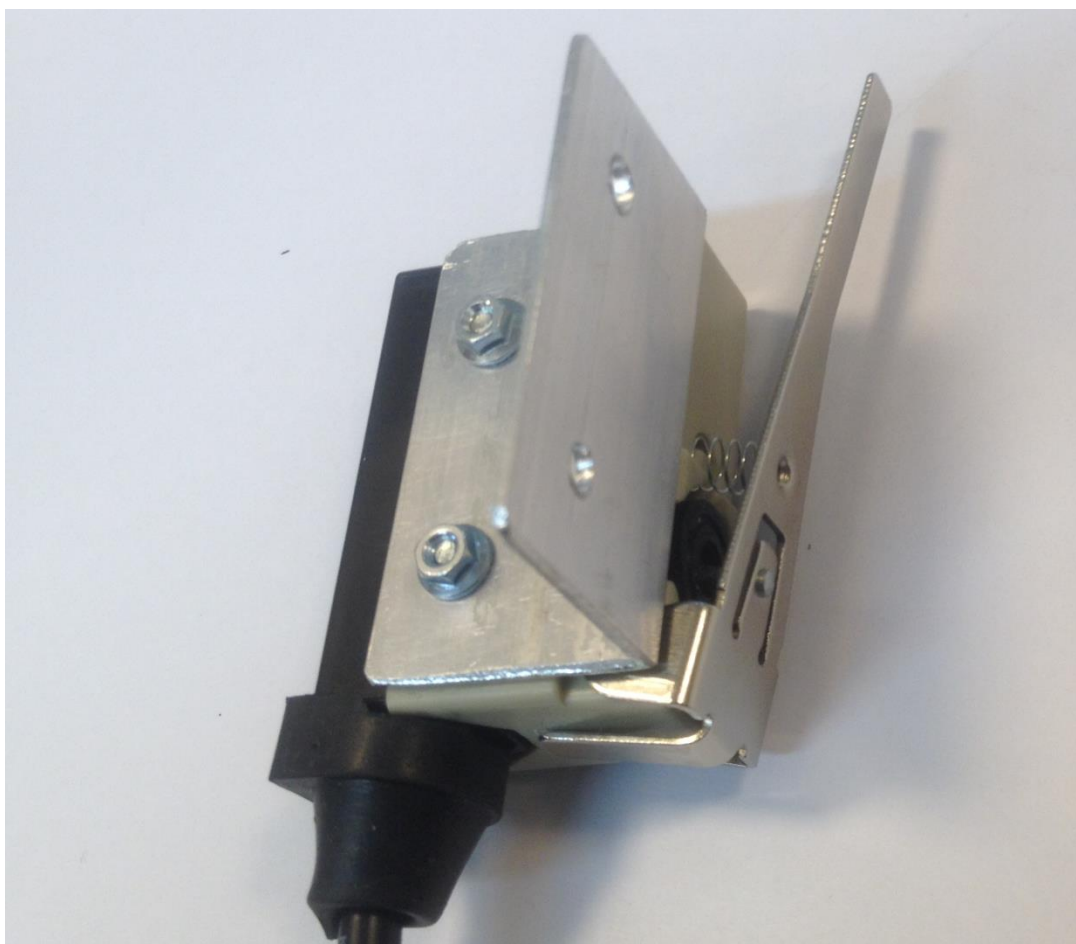
Рис.3.3.7-1 Присоединяем уголок к Датчику вскрытия.
