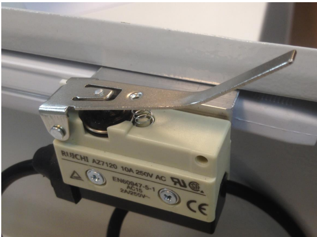
Рис.3.3.10-1 Регулировка положения коромысла выключателя.
