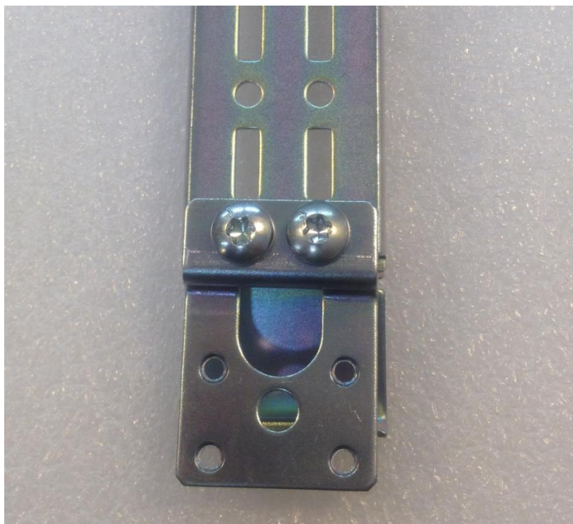
Рис.3.4.8-1 Присоединение удлинителя к шине внутреннего монтажа
