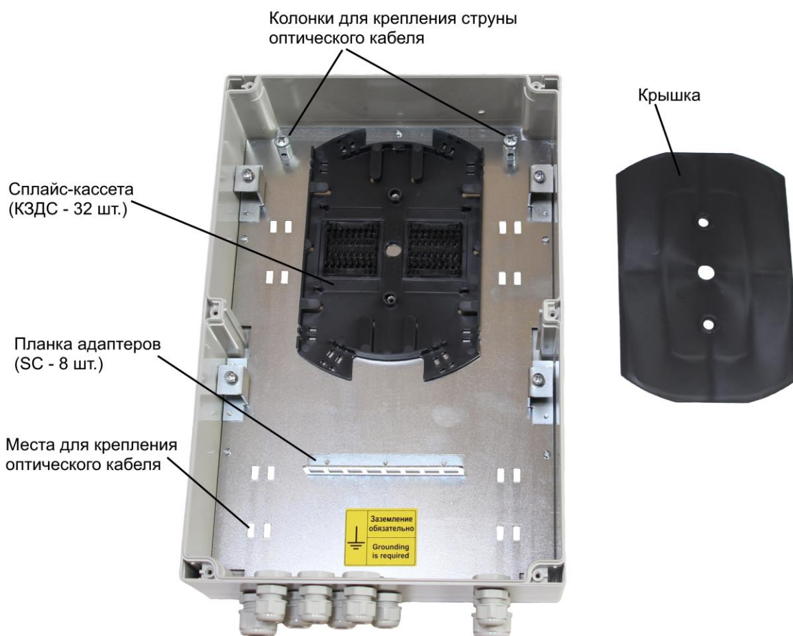
Рисунок 3.4 - Оптический кросс
