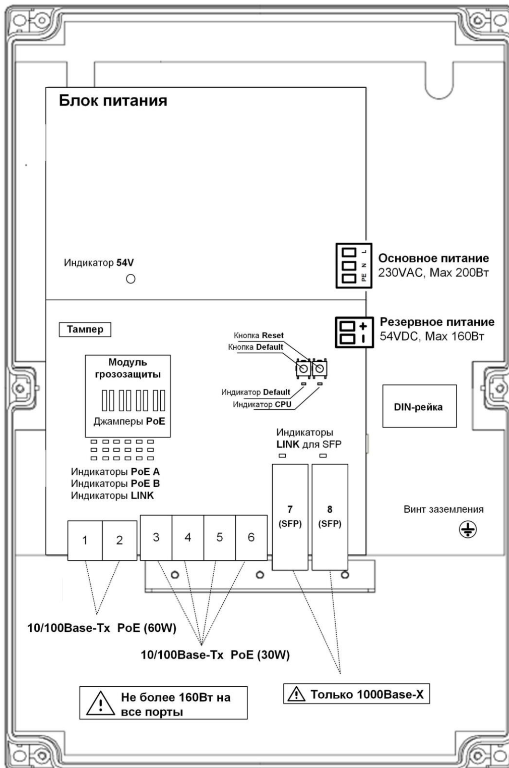
Рисунок 3.2 - Расположение элементов коммутатора PSW -2G6F+
