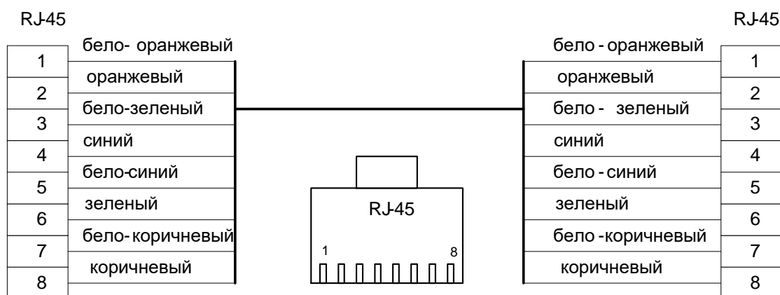
Рисунок 7.6 - Разделка кабеля.
