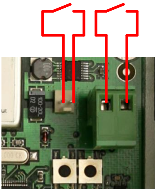
Рисунок 3.6 - Сухие контакты
