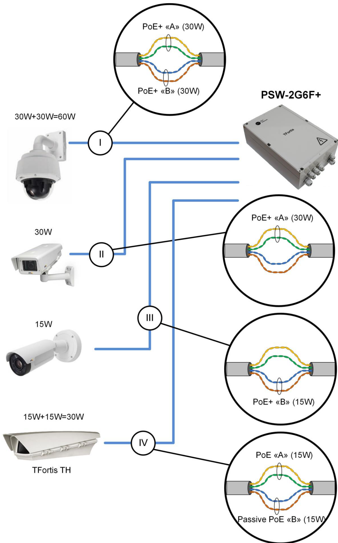
Рисунок 3.3 - Схема питания по PoE для разных случаев
