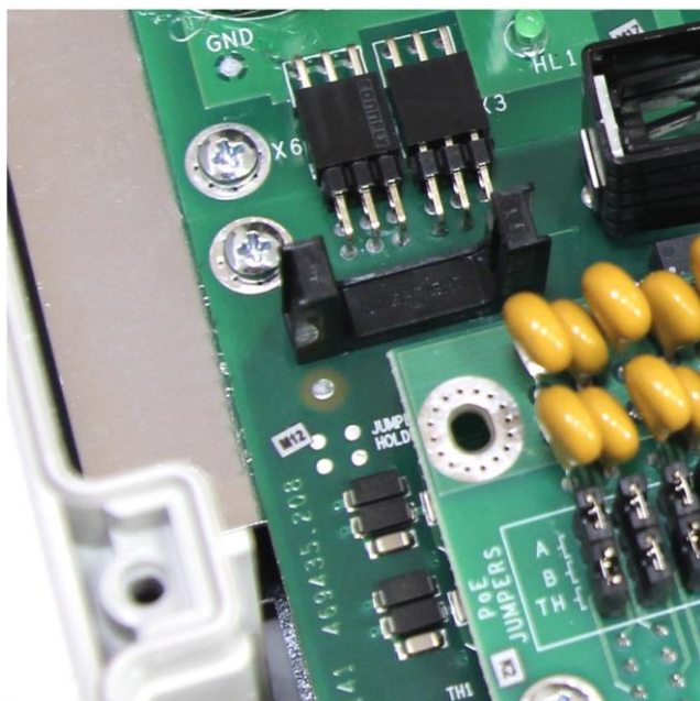
Рисунок 3.5.1 - Датчика вскрытия на плате
