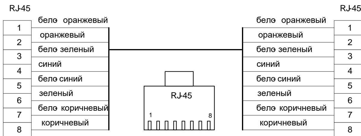
Рисунок 7.4 - Разделка кабеля.
