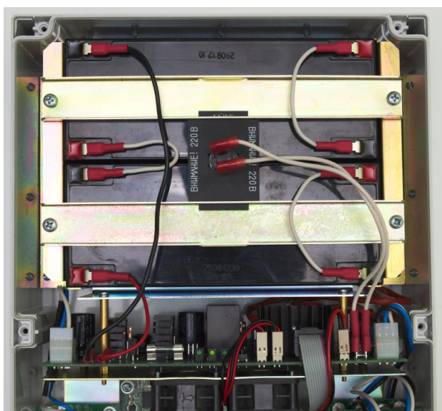
Рисунок 3.9.5 - Подключение АКБ.
