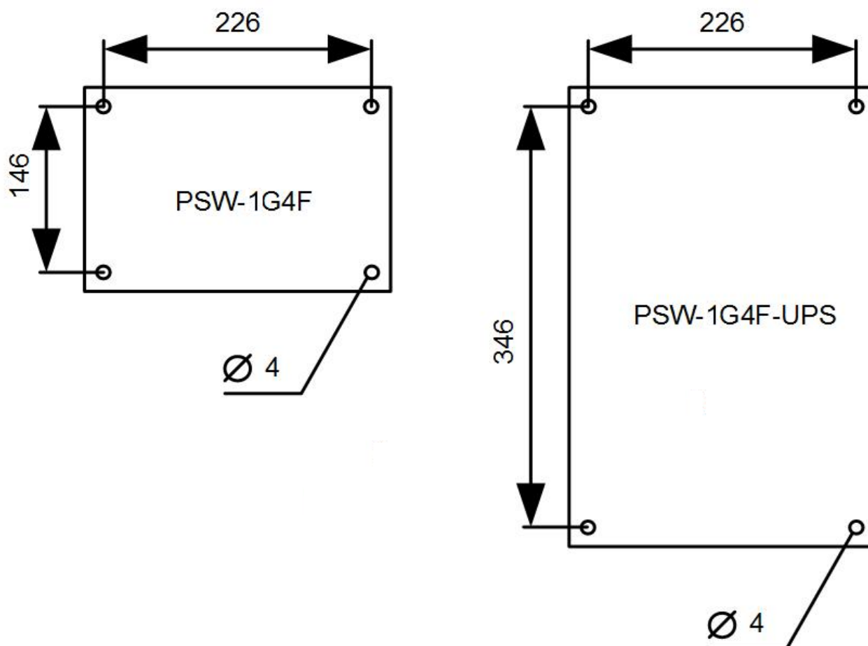
Рисунок 7.1.1 - Разметка крепления
