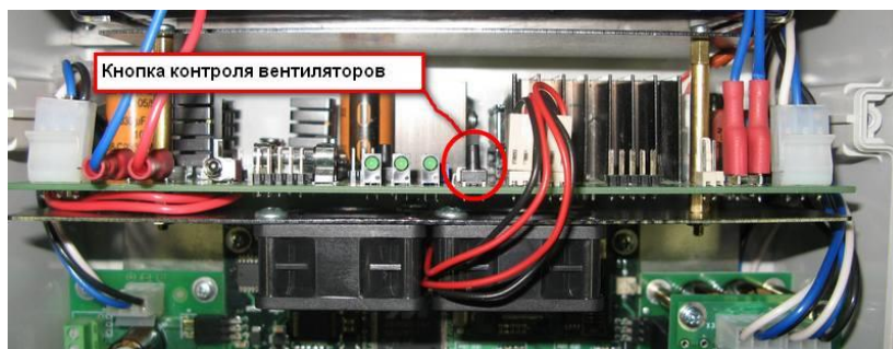
Рисунок 3.9.6 - Проверка работоспособности вентиляторов.
