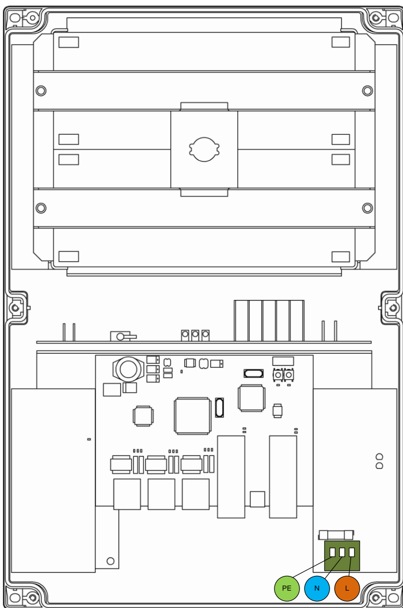
Рисунок 7.3.2 - Подключение питания к PSW-1G4F-UPS.
