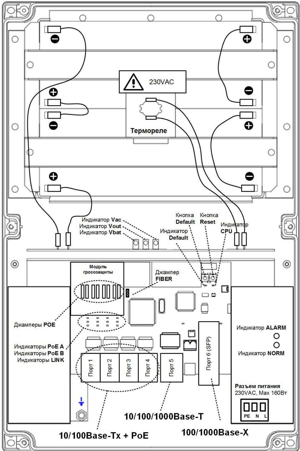
Рисунок 3.2.2 - Расположение элементов PSW -1G4F-UPS
