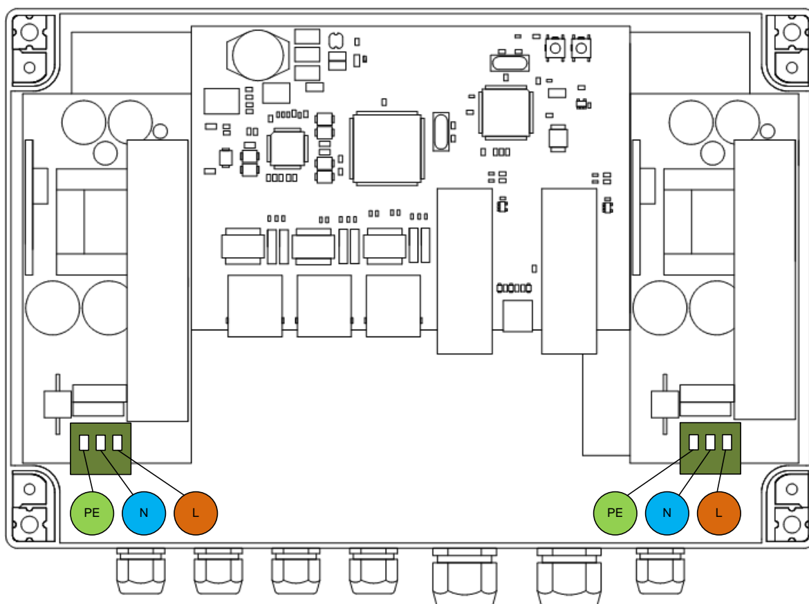
Рисунок 7.3.1 - Подключение питания к PSW-1G4F.
